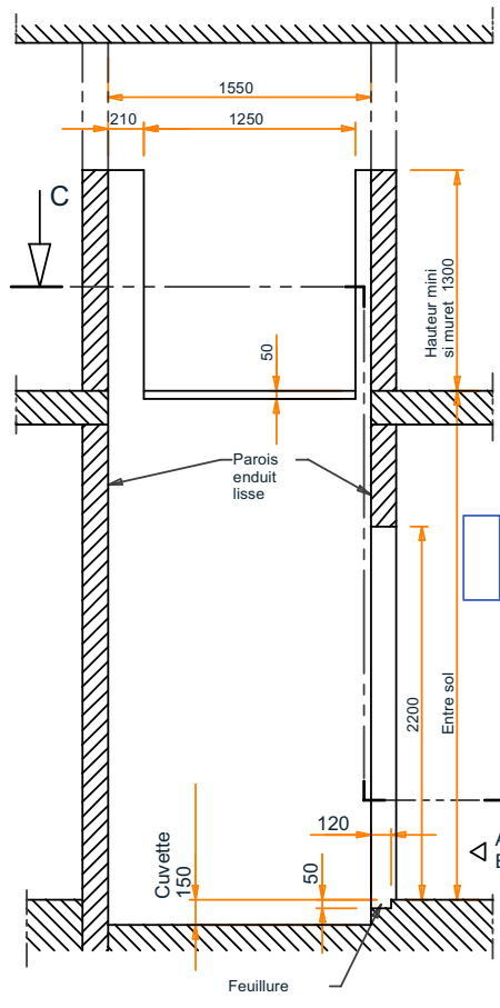
COUPE BB
