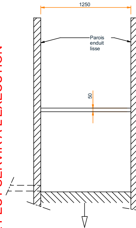
COUPE BB
